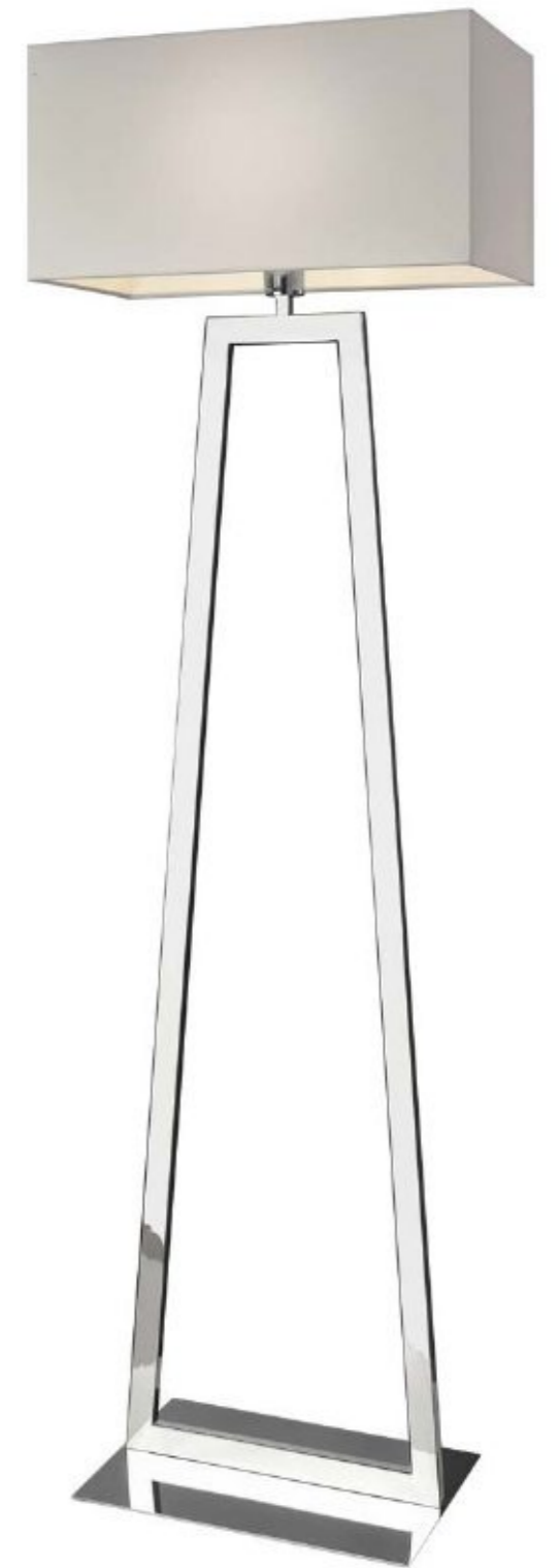
LYON | 96640 h 152 cm, schirm 25 x 48 cm max. 60 W, 230 V, E27 stehleuchte, edelstahl poliert, stoffschirm weiß floor lamp, stainless steel polished, white fabric shade lampdaire, lacier inoxydable polit, abat-jour tissu blanc
